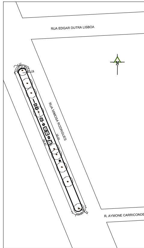
PLANTA BAIXA - ACADEMIA DE RUA COTADA RUA MIMOSA RODRIGUES TRECHO 02
