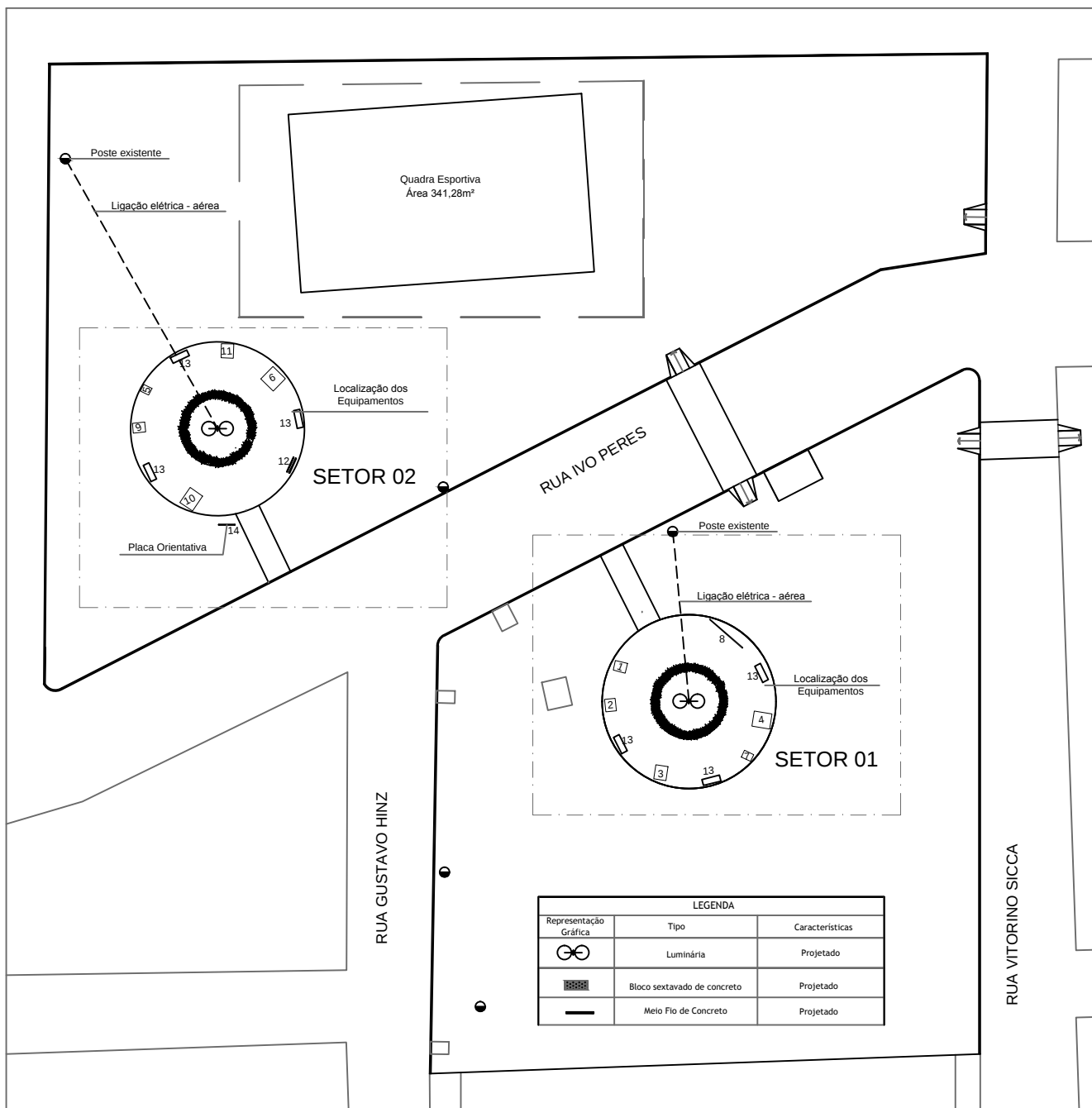
PLANTA BAIXA COTADA
