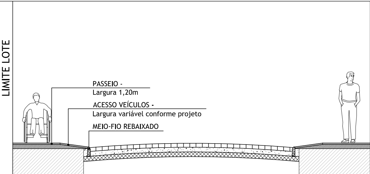
SEÇÃO TRANSVERSAL ACESSO VEÍCULOS SEM ESCALA
