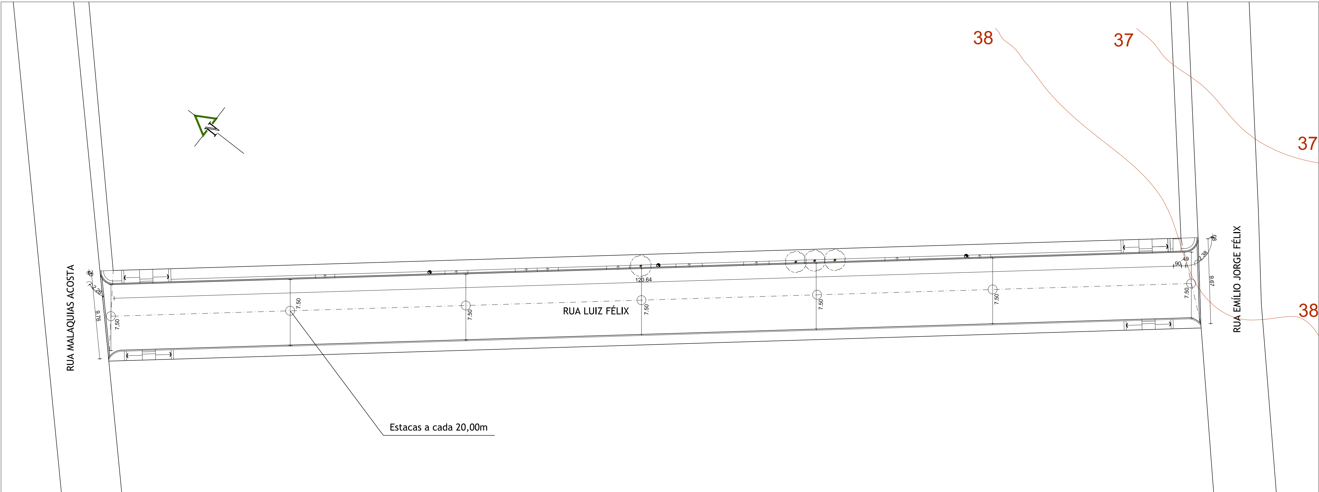
PLANTA BAIXA DE MEIO-FIO - COTADA RUA LUIZ FÉLIX ESC.:1/250
