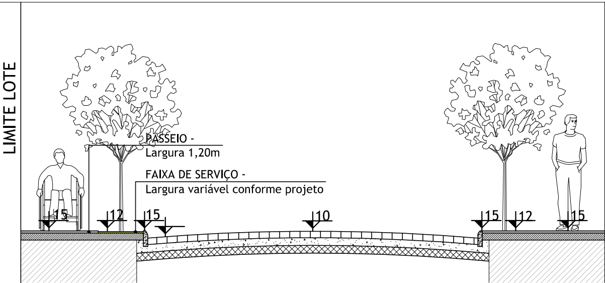
SEÇÃO TRANSVERSAL PASSEIOS SEM ESCALA
